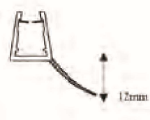
04800250 Burlete ala lateral abierta 6-8mm
