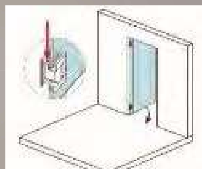
8060 Bisagra lateral hidráulica. Especial hermética
